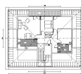
PLAN DES COMBLES
