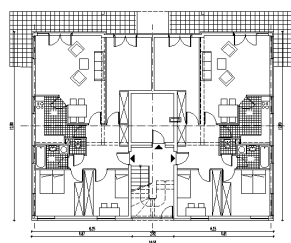
PLAN DU RDC
