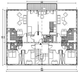
PLAN DU 1ER ETAGE
